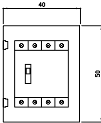
GABINETE CON INTERRUPTOR TETRAPOLAR COINCIDENTE CON EL COMPARTIMIENTO DE BARRAS
