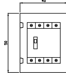
GABINETE CON INTERRUPTOR TETRAPOLAR COINCIDENTE CON EL COMPARTIMIENTO DE BARRAS
